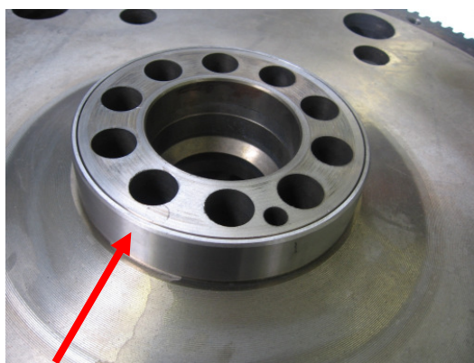
Маховик с вращающимся кольцом
