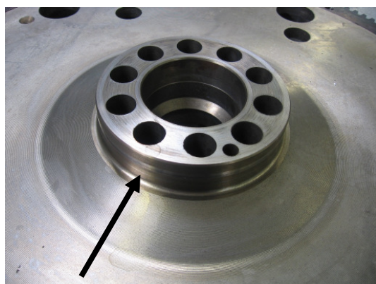
Маховик без вращающегося кольца
