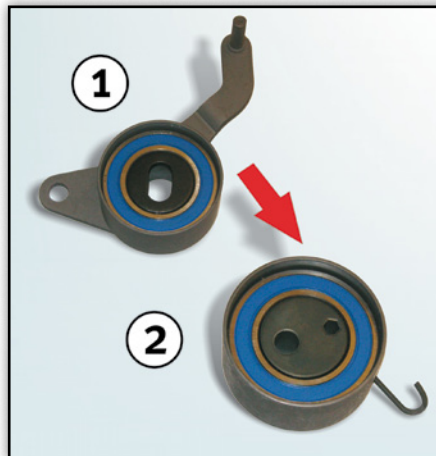
Bild 1: Ersetzte Spannrolle 531 0166 20 (1) und Nachfolger 531 0819 10 (2)
