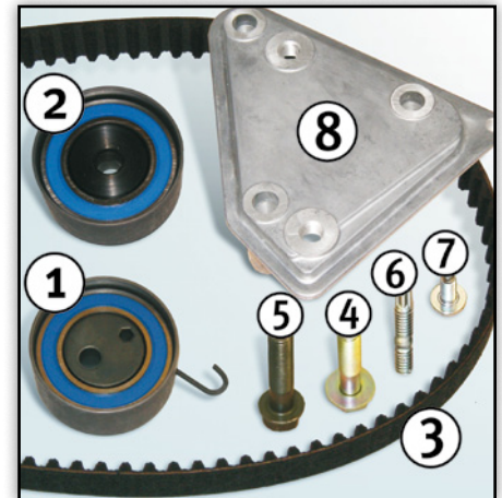
Bild 2: Verpackungsinhalt 530 0492 10
