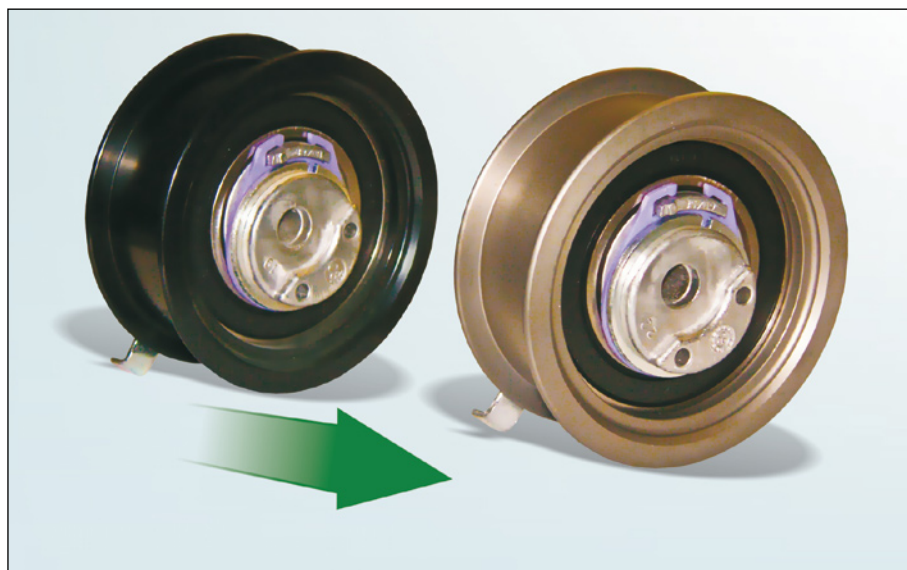
Bild 1: Verbesserte Beschichtung der Laufbahn - hier exemplarisch dargestellt an der Artikel-Nr. 531 0524 30
