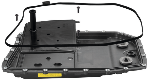
ÖLWANNE INKL. WECHSELFILTER UND DICHTUNG OILPAN INCL. FILTER SET AND SEALING
