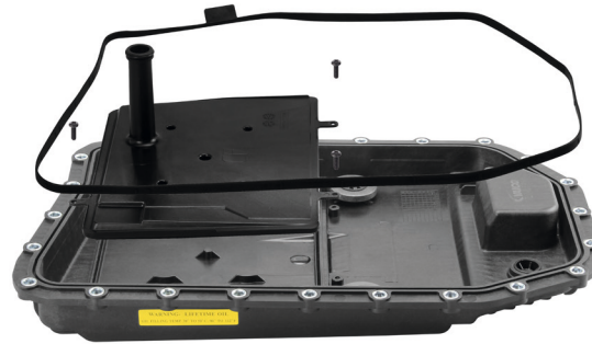
ÖLWANNE INKL. WECHSELFILTER UND DICHTUNG OILPAN INCL. FILTER SET AND SEALING
